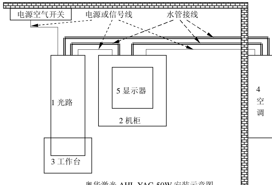
奥华激光 AHL-YAG-50W 安装示意图
